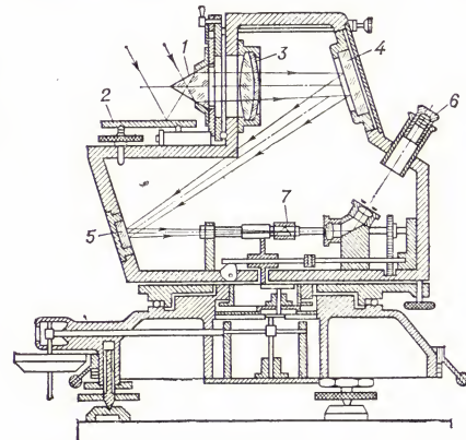
Призменная астролябия Данжона: 1 — призма перед объективом; 2 — ртутный горизонт; 3 — объектив; 4—5 — зеркала; 6 — окуляр; 7 — двойная призма Воластона.
